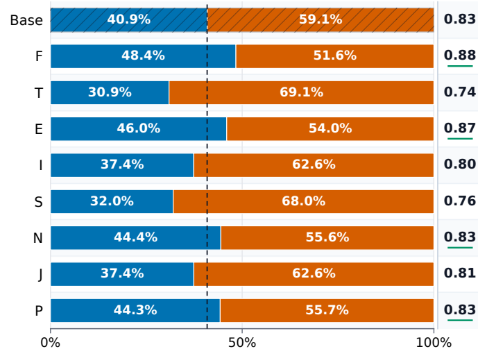
Llama-3.2-3B
